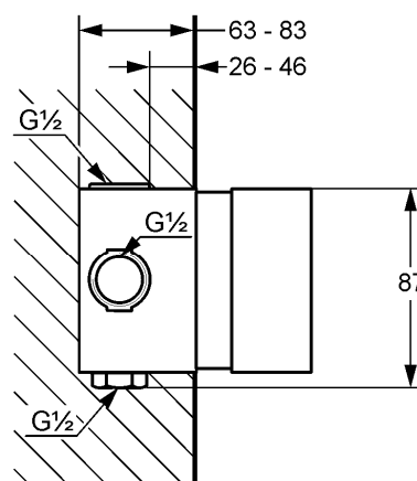
Maßzeichnung II
