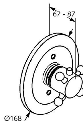
Maßzeichnung I
