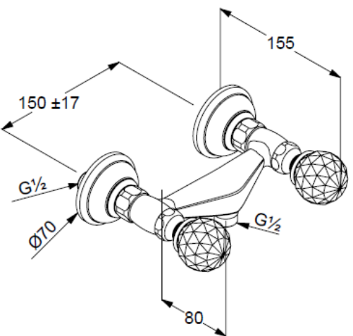
Maßzeichnung
