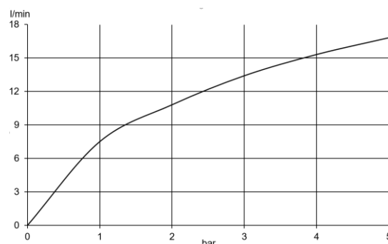
Durchflussdiagramm
