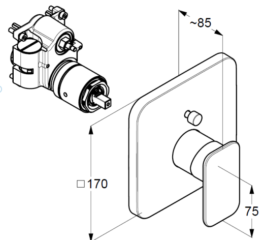
Maßzeichnung
