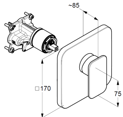
Maßzeichnung
