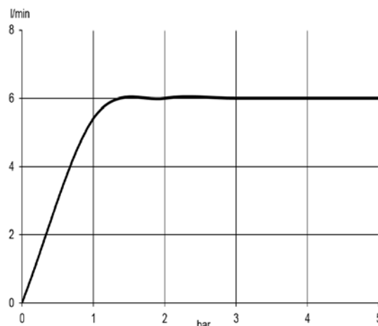
Durchflussdiagramm
