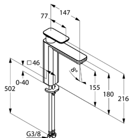
Maßzeichnung
