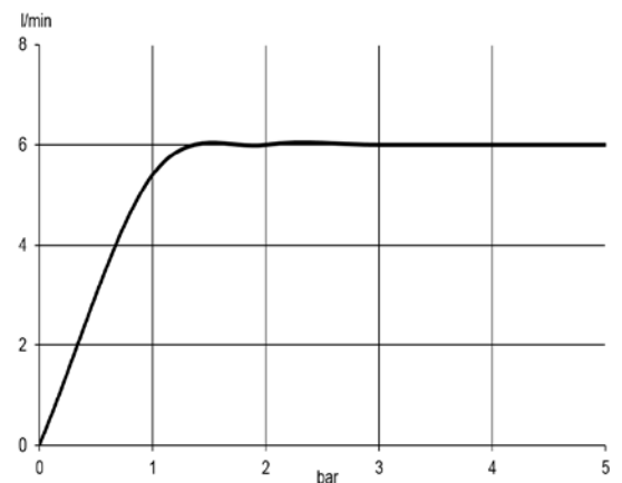
Durchflussdiagramm
