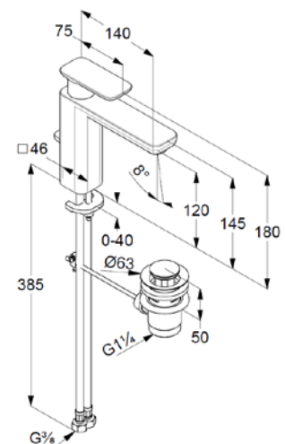
Maßzeichnung
