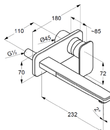
Maßzeichnung
