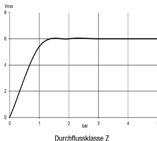
Durchflussdiagramm
