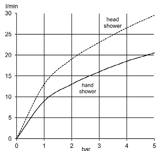
Durchflussdiagramm
