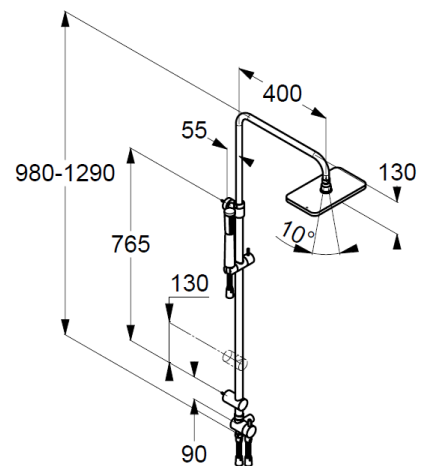
Maßzeichnung
