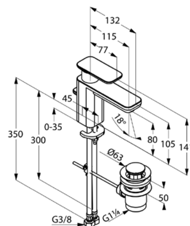
Maßzeichnung
