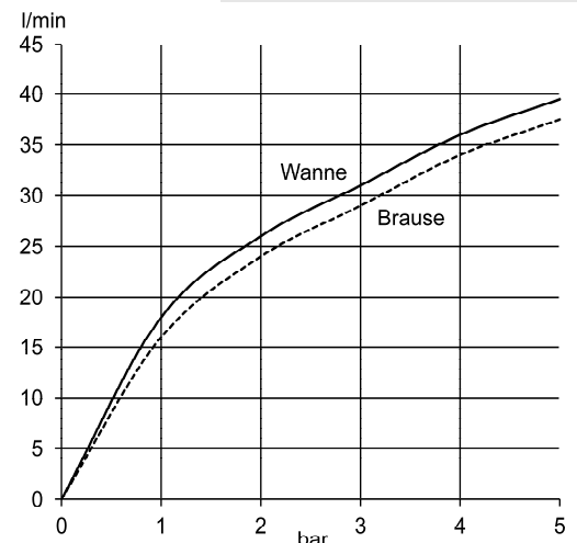
Durchflussdiagramm
