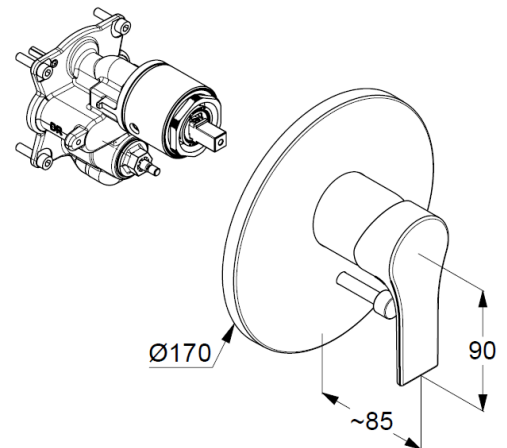
Maßzeichnung
