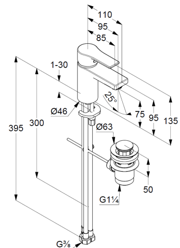
Maßzeichnung
