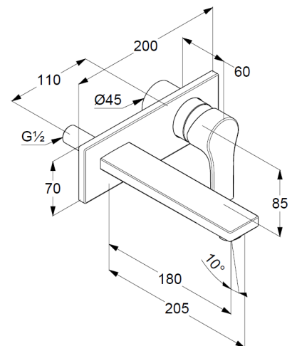
Maßzeichnung
