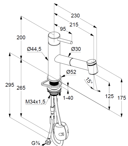
Maßzeichnung
