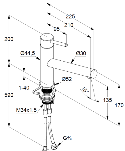
Maßzeichnung
