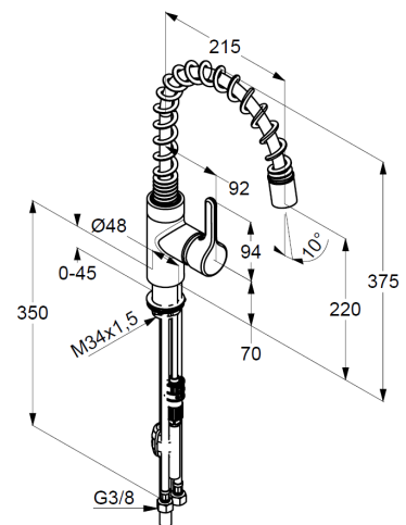
Maßzeichnung
