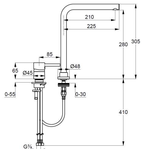
Maßzeichnung
