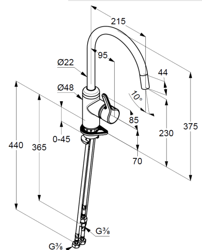
Maßzeichnung
