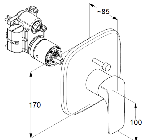
Maßzeichnung
