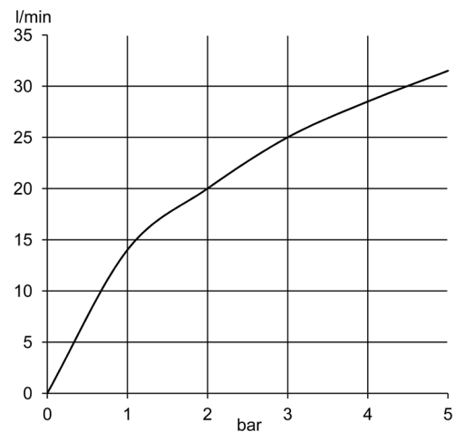
Durchflussdiagramm
