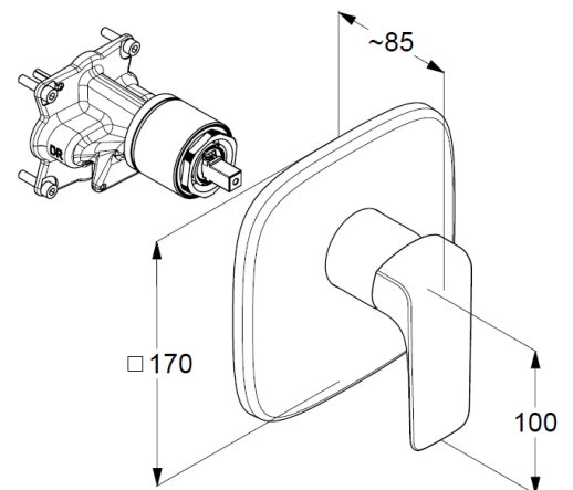
Maßzeichnung
