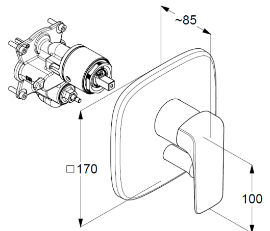
Maßzeichnung
