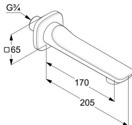
Maßzeichnung
