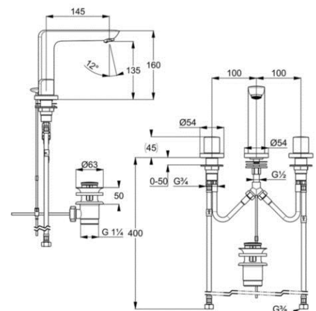
Maßzeichnung
