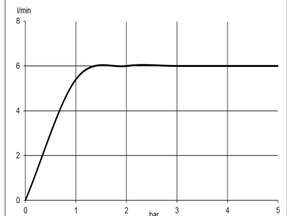
Durchflussdiagramm
