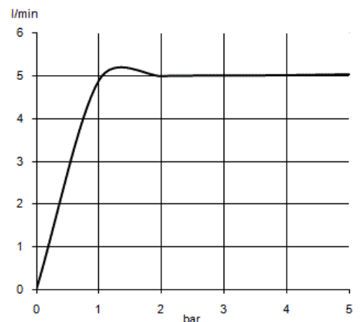
Durchflussdiagramm
