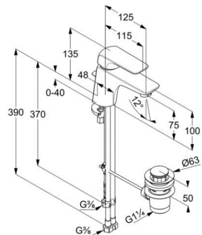
Maßzeichnung
