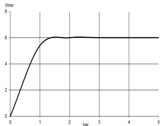
Durchflussdiagramm
