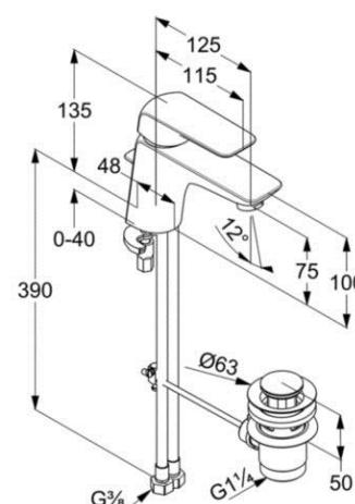
Maßzeichnung
