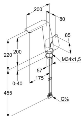
Maßzeichnung
