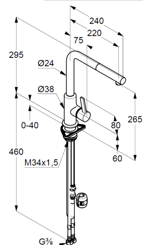
Maßzeichnung
