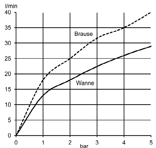
Durchflussdiagramm
