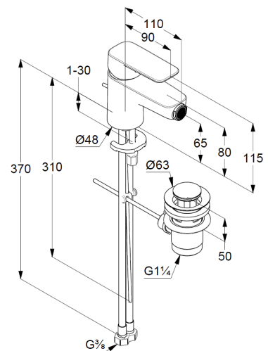
Maßzeichnung
