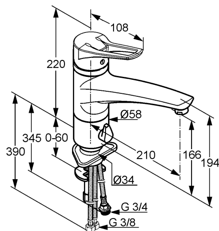
Maßzeichnung
