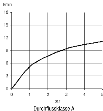
Durchflussdiagramm
