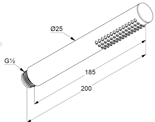
Maßzeichnung
