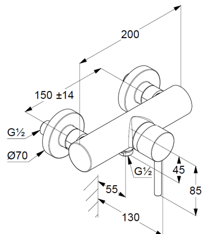
Maßzeichnung
