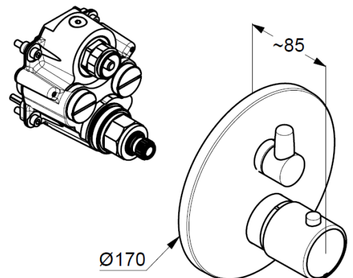
Maßzeichnung
