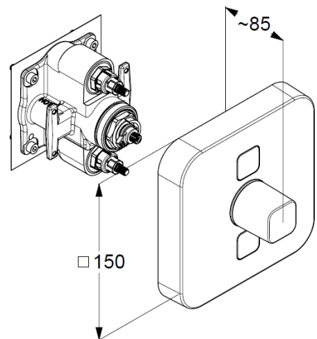
Maßzeichnung
