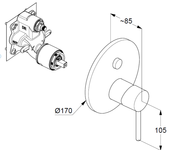
Maßzeichnung
