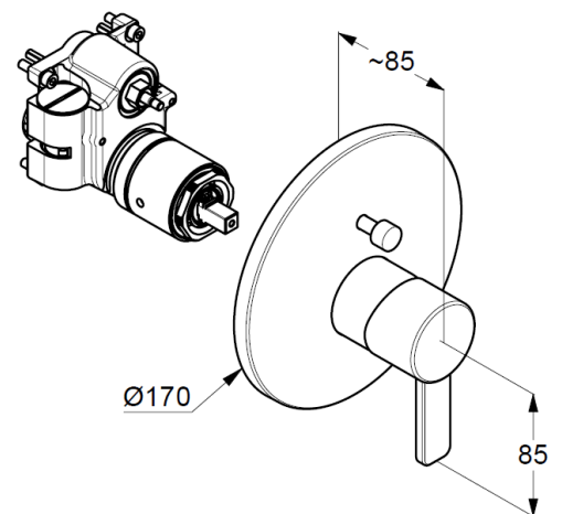
Maßzeichnung
