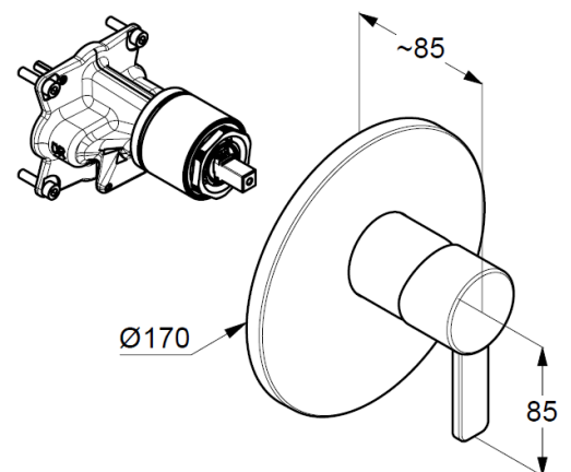
Maßzeichnung
