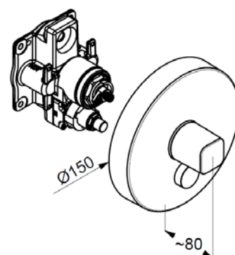
Maßzeichnung
