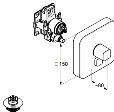
Maßzeichnung
