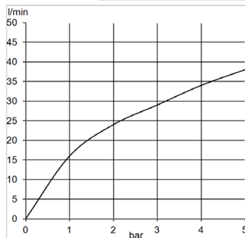
Durchflussdiagramm
