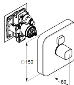
Maßzeichnung
