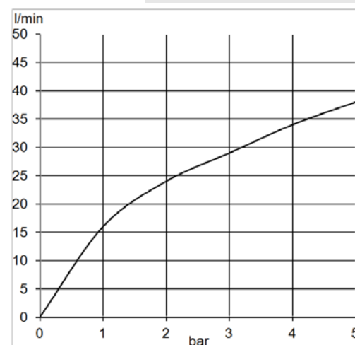
Durchflussdiagramm
