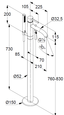
Maßzeichnung
