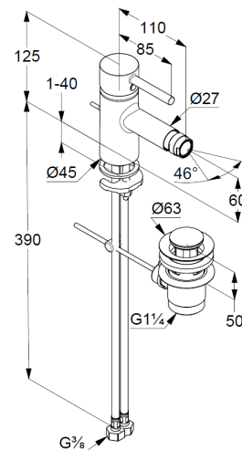
Maßzeichnung
