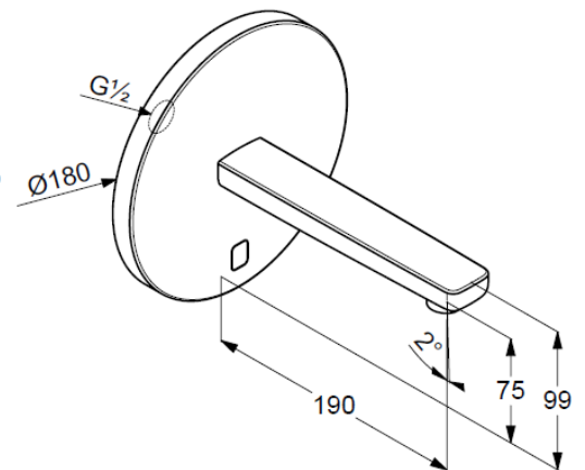
Maßzeichnung
