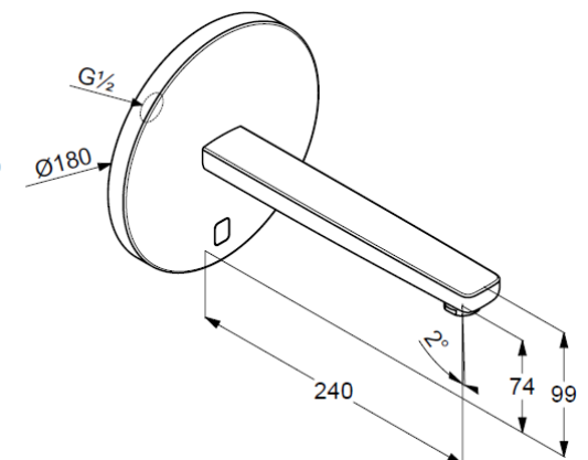
Maßzeichnung
