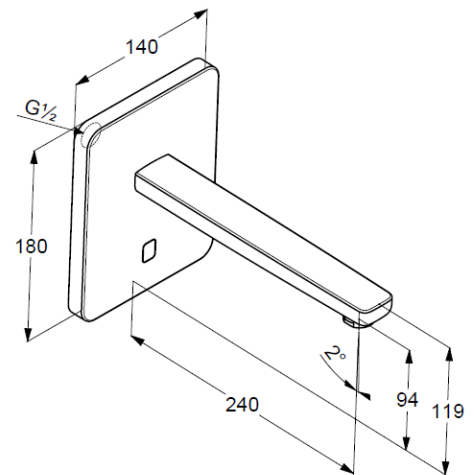
Maßzeichnung
