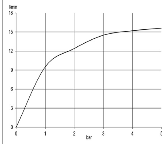
Durchflussdiagramm
