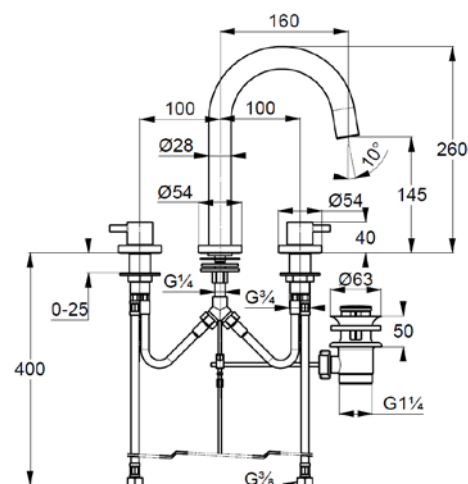
Maßzeichnung
