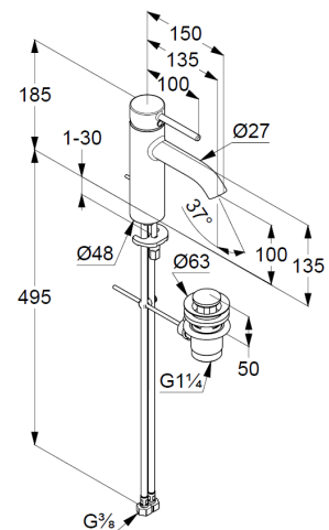
Maßzeichnung
